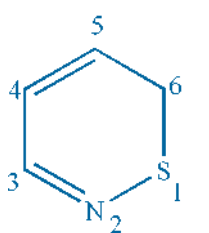
1,2-Thiazine
