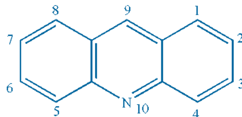
Acridine
