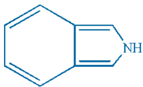
Isoindole
