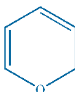
\alpha -Pyrrones
