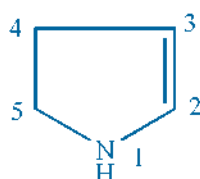
\Delta^2 -Pyrroline
