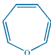
Oxepine
