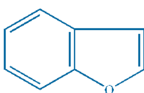
Benzofuran
