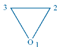
Oxirane
