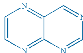
Pteridine
