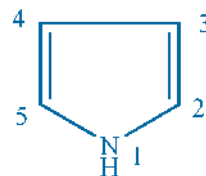
Pyrrole
