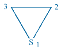
Thiirane
