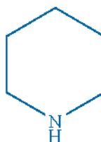
Piperidine
