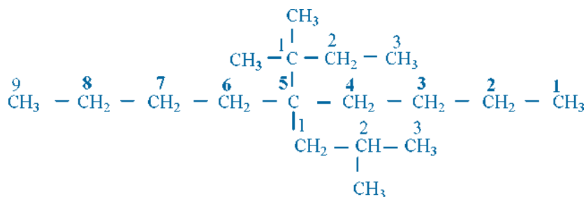
5-(1,1-Dimethylpropyl)-5-(2-methylpropyl) nonane
