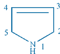
\Delta^3 -Pyrroline
