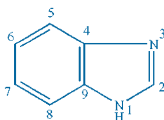
Benzimidazole
